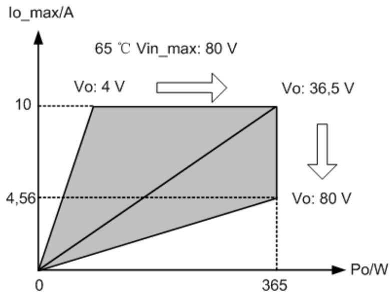
Figura A-3 Curva di relazione I_{o\_max} - P_o ( 65\text{ }^\circ\text{C} , V_{in\_max} = 80\text{ V} )
