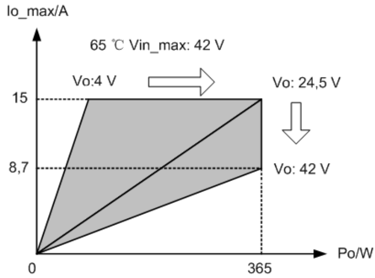
Figura A-2 Curva di relazione I_{o\_max} - P_o ( 65\text{ }^\circ\text{C} , V_{in\_max} = 42\text{ V} )
