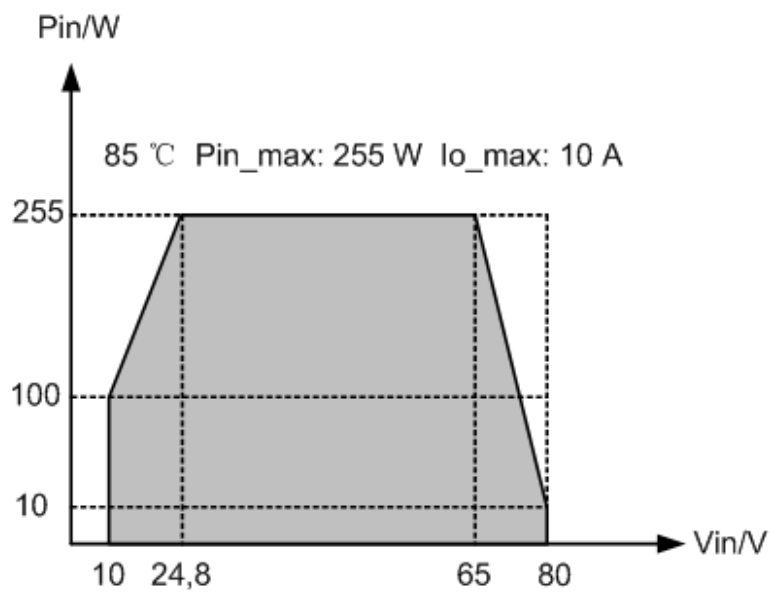
Figura A-5 Curva di relazione P_{in} - V_{in} ( 85\text{ }^\circ\text{C} , P_{in\_max} = 255\text{ W} , I_{o\_max} = 10\text{ A} )
