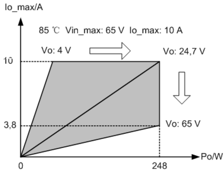
Figura A-4 Curva di relazione I_{o\_max} - P_o ( 85\text{ }^\circ\text{C} , V_{in\_max} = 65\text{ V} , I_{o\_max} = 10\text{ A} )
